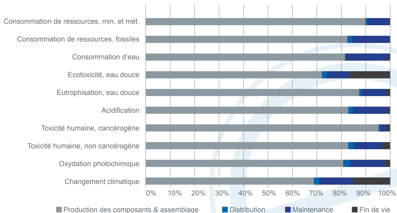
Figure 2 : répartition des impacts environnementaux de la pompe doseuse D6 (2%)
