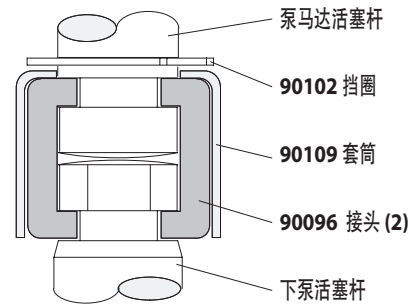
泵连接详图
