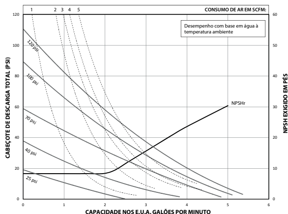
PD01P-XXS-XXX 1/4" "BOMBA DE DIAFRAGMA NÃO METÁLICA
