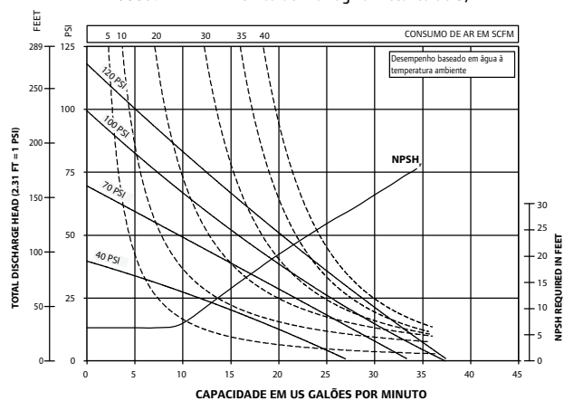
66607X-XXX -A Bomba de Diafragma Metálica de 3/4"
