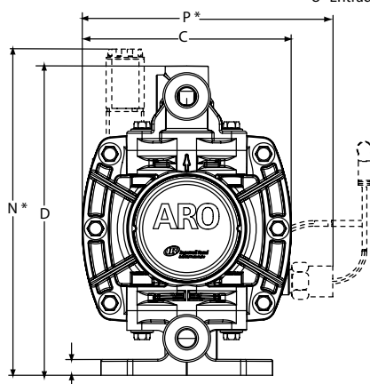
PD01P-XXS-XXX 1/4" "BOMBA DE DIAFRAGMA NÃO METÁLICA
