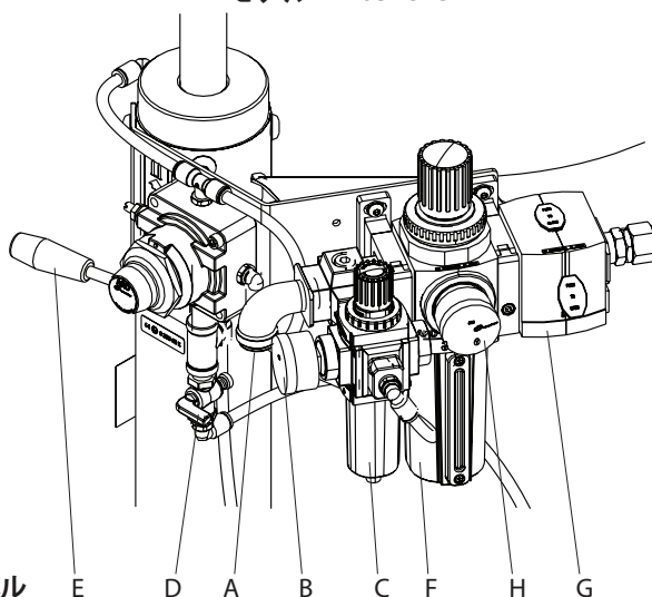
フォロワープレート空気供給バルブ
