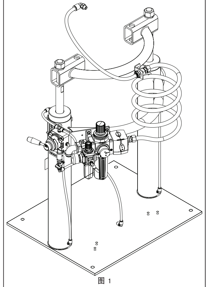
RM052S-XXX-XX 双柱升降机/冲压机
