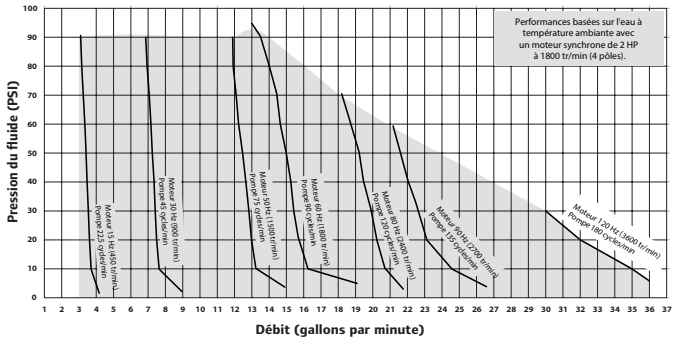
Pression de sortie maximale de 190 PSIG (13,1 bar) de la E2P10-XXXXX-CX-XXA. La conception de la tuyauterie de l'utilisateur final doit être évaluée pour résister à cette pression.
