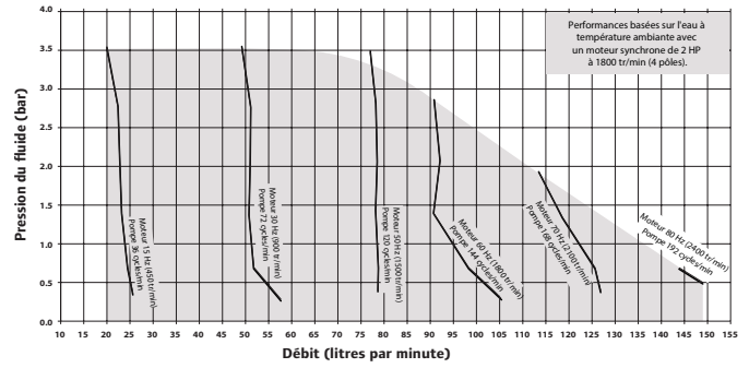
Pression de sortie maximale de 100 PSIG (6,89 bar) de la E2P10-XXXXX-AX-XXA La conception de la tuyauterie de l'utilisateur final doit être évaluée pour résister à cette pression.
