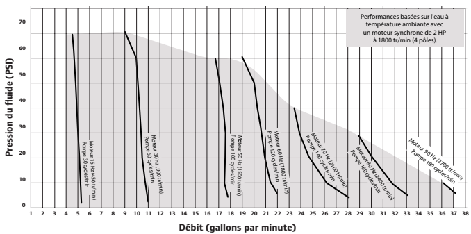
Pression de sortie maximale de 140 PSIG (9,65 bar) de la E2P10-XXXXX-BX-XXA La conception de la tuyauterie de l'utilisateur final doit être évaluée pour résister à cette pression.
