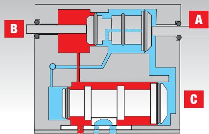
Von links nach rechts bewegende Membran
