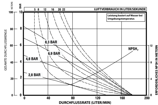
LEISTUNGSKURVE 6661XX-XXX-C NICHTMETALLISCHE 1"-MEMBRANPUMPE
