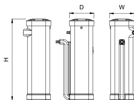
Ecosep 25 - Ecosep 35
