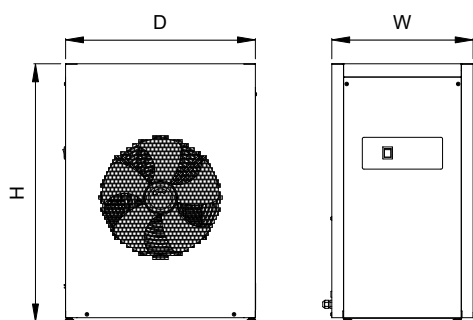
HTD 35 - HTD 170
