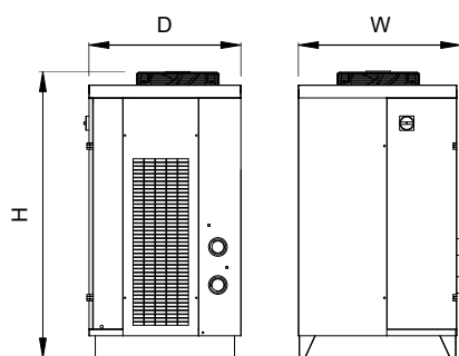
ED 600 - ED 1000
