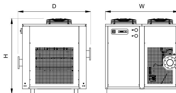
ESD 5300 - ESD 6000
