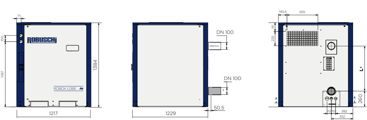
Robox Lobe ES-2.0
