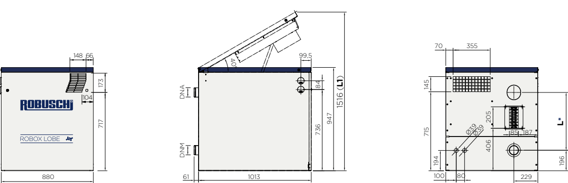
Robox Lobe ES-1.5
