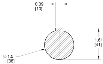
SECTION A-A SCALE 1.000
