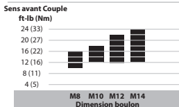
Figure B — Serré à l'aide d'une clé
