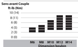
Figure A — Serré à la main
