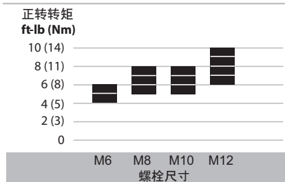
图A— 手动拧紧
