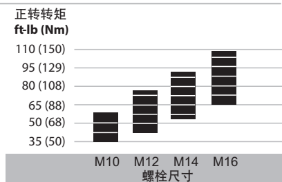
图B— 扳手拧紧
