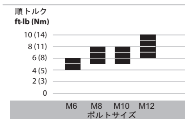
図A— ② 手による締め付け
