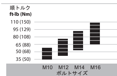
図B— ② 手による締め付け
