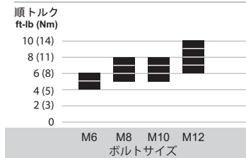
図 A 手による締め付け
