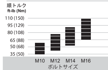
図 B 手による締め付け
