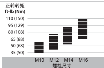
图B — 扳手拧紧
